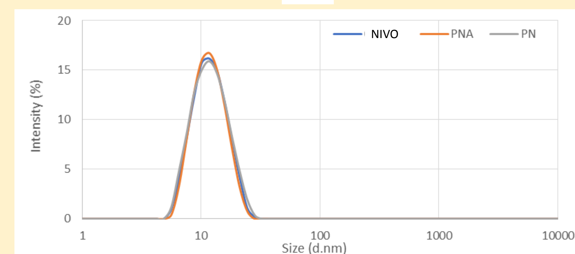
DLS
