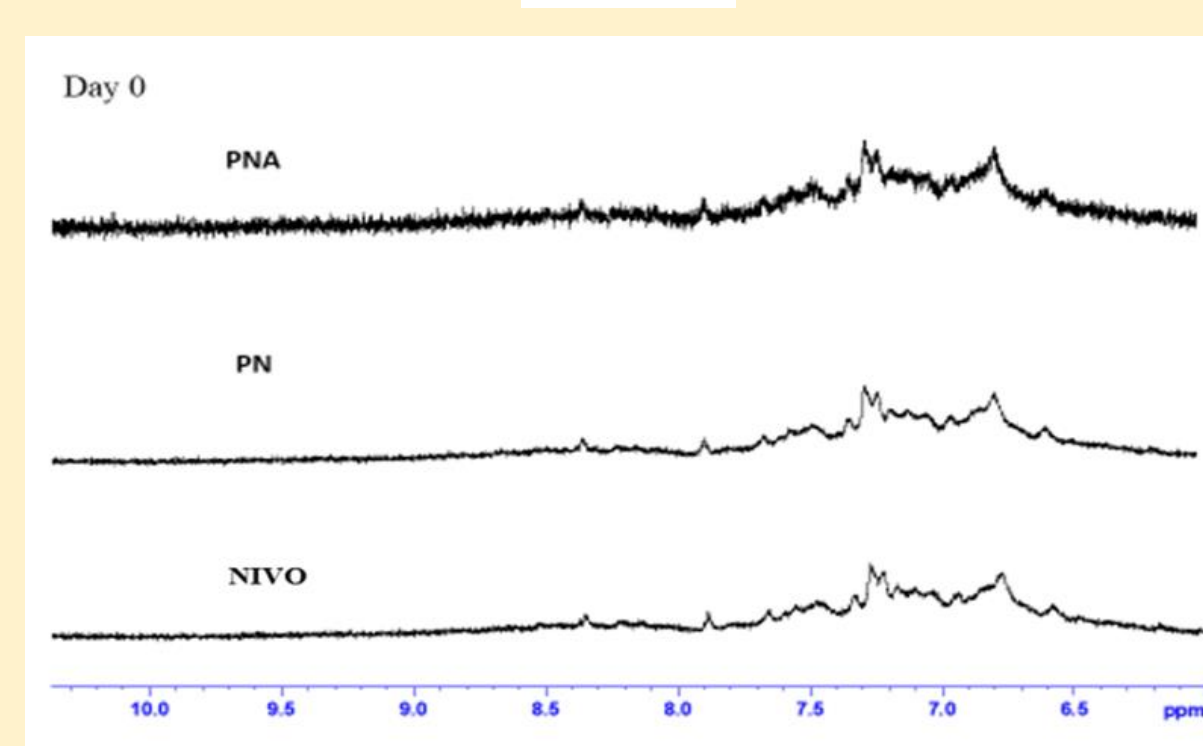
NMR
