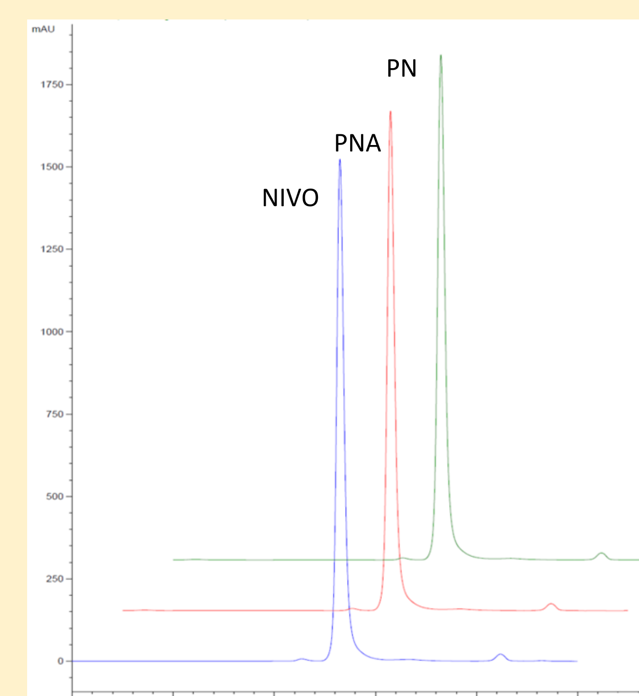
DLS
